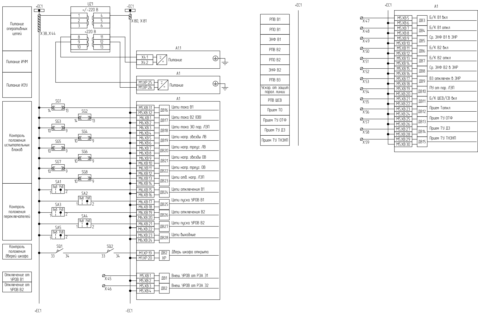
Рисунок В.2 – Схема электрическая принципиальная (часть 2)
