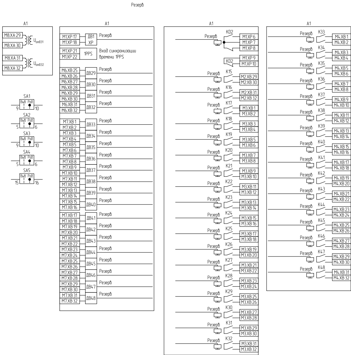
Рисунок В.4 – Схема электрическая принципиальная (часть 4)
